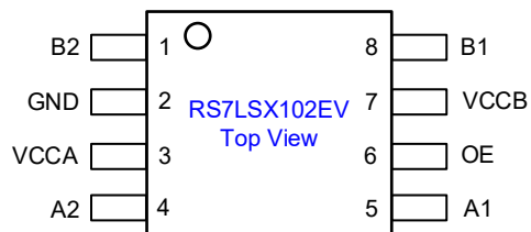
VSSOP8 (Top view)
