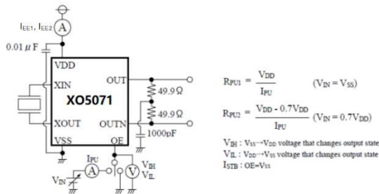
Measurement Circuit 1: I EE1 , I EE2 , V IH , V IL , R PU1 , R PU2
